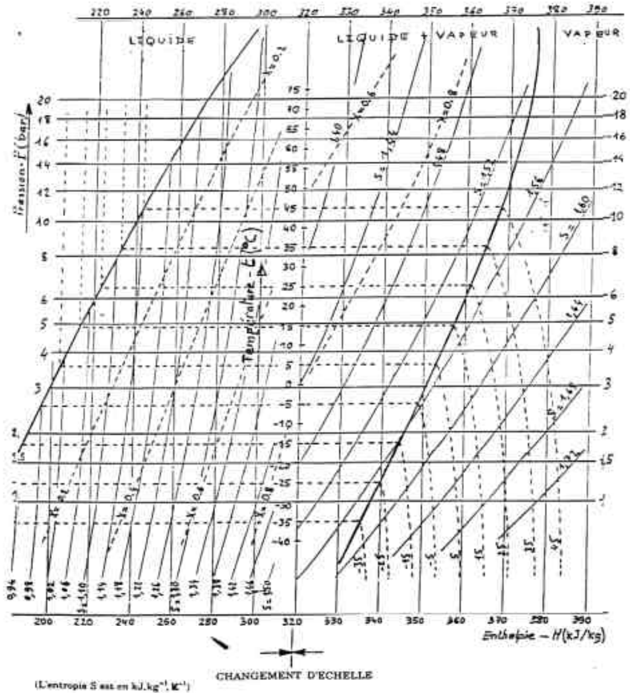
Diagramme Enthalpie-Pression du fréon
